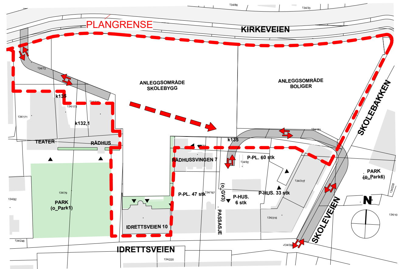
FASE 2 - byggefase med midlertidig adkomst for eksisterende bebyggelse
